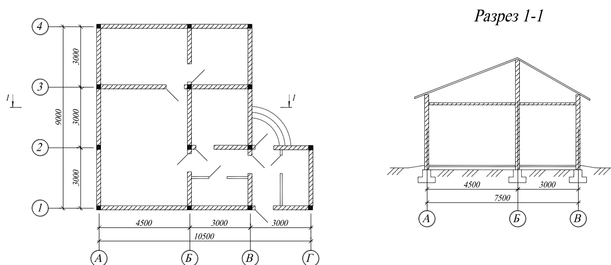
Рисунок 1- Конструктивная схема жилого дома
