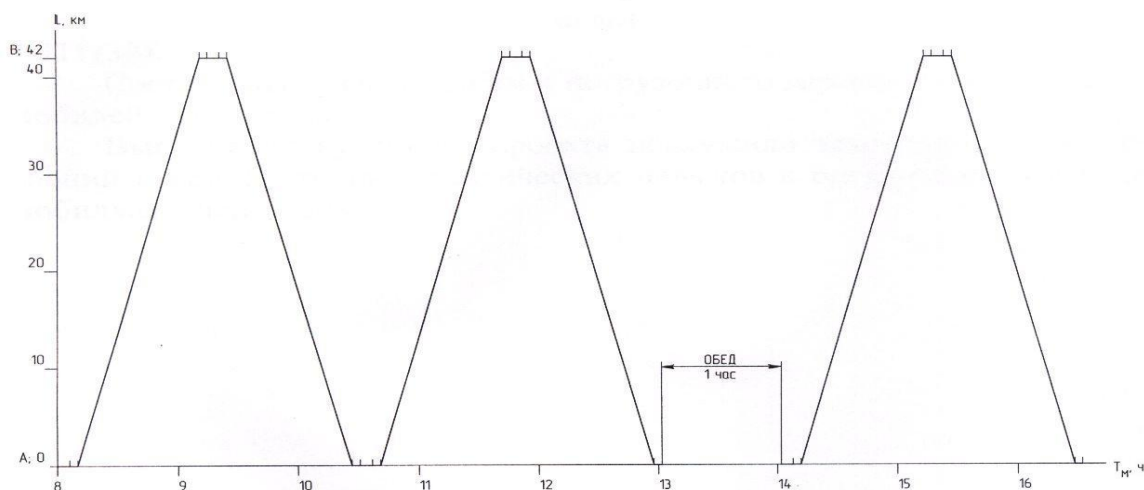
Рисунок 10.1 - График работы автомобиля на маятниковом маршруте
